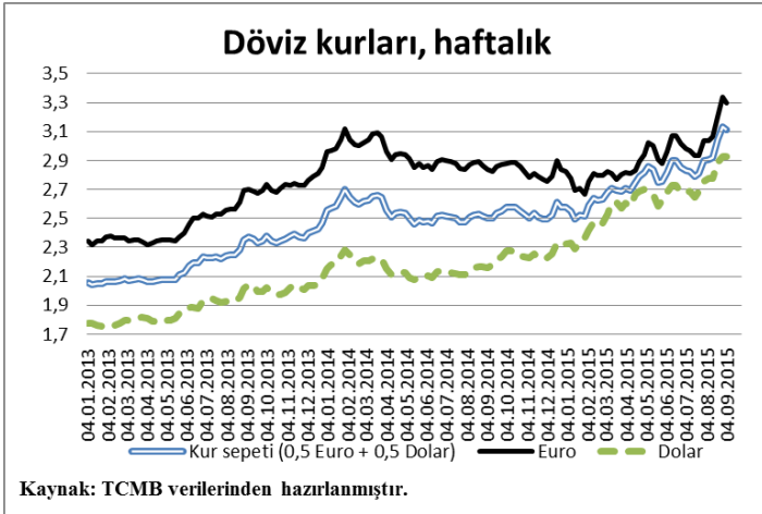
Şekil 2: Haftalık Döviz Kurları (Ocak 2013 – Eylül 2015)
